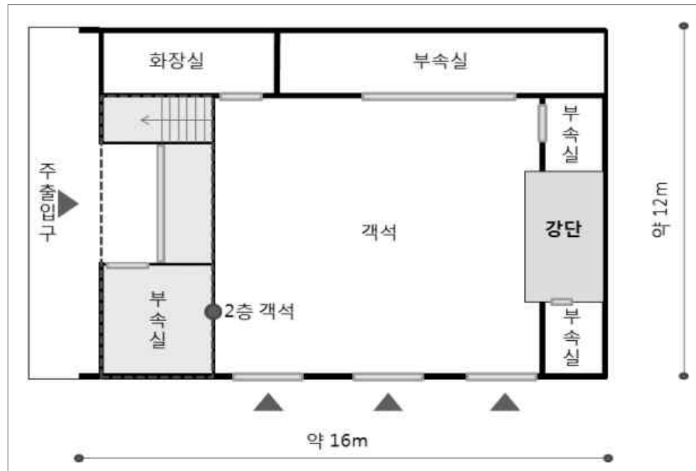
대성동 공회당 '자유의 집' 약실측 평면도
